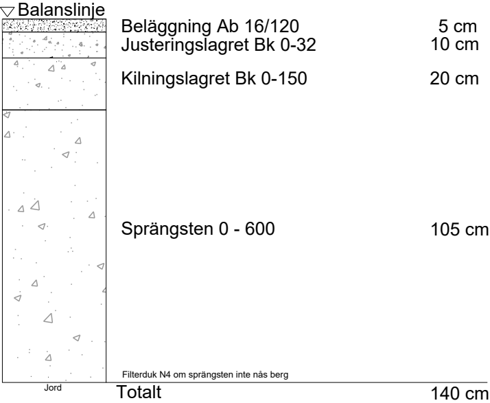
Konstruktionprofil B, 1:20, sprängstenbank
