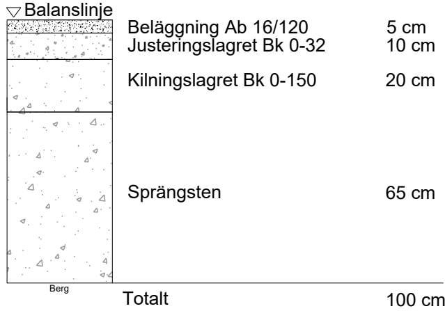
Konstruktionprofil A, 1:20, lösbrytning, -1,0 m av balanslinje
